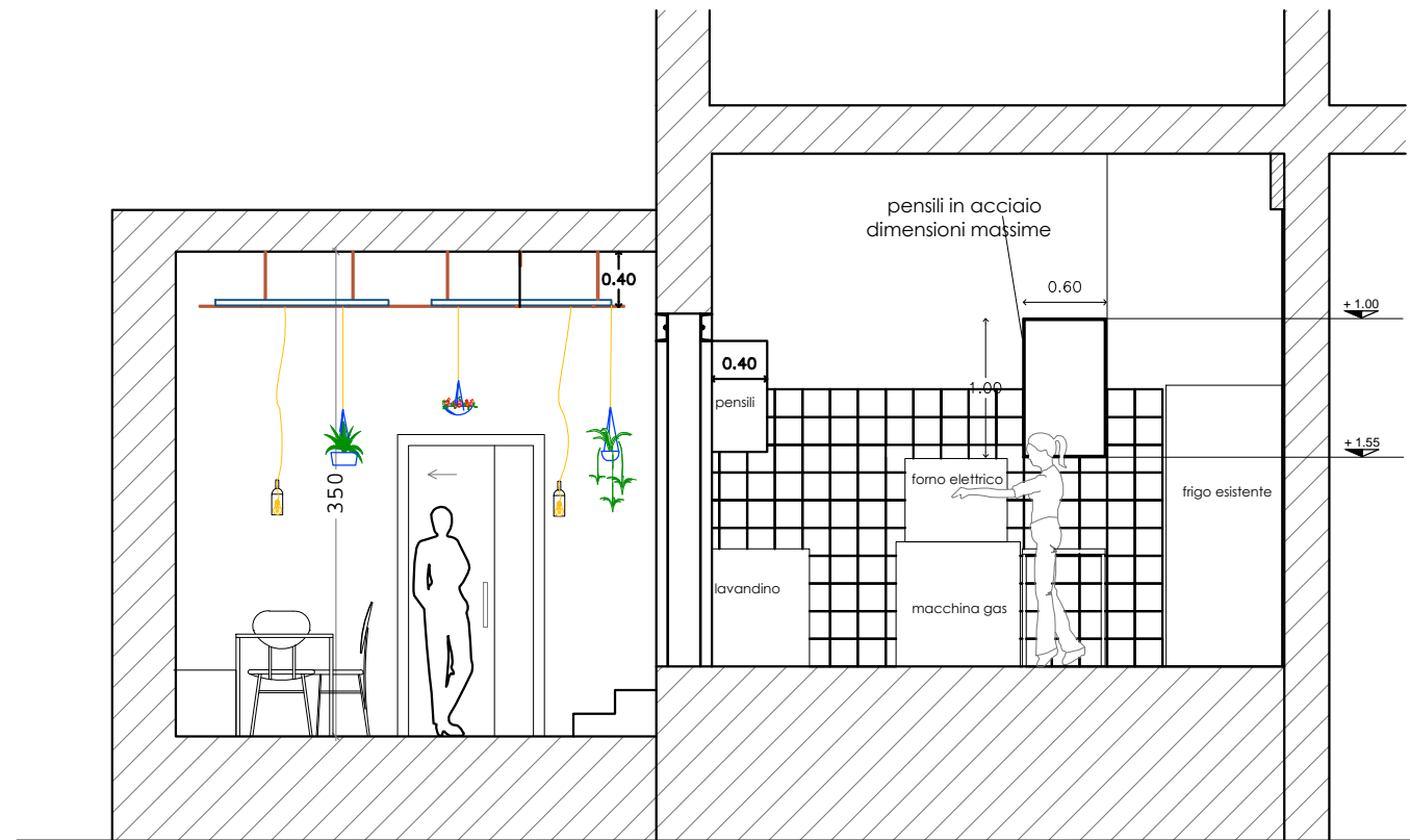
PROSPETTO AA
