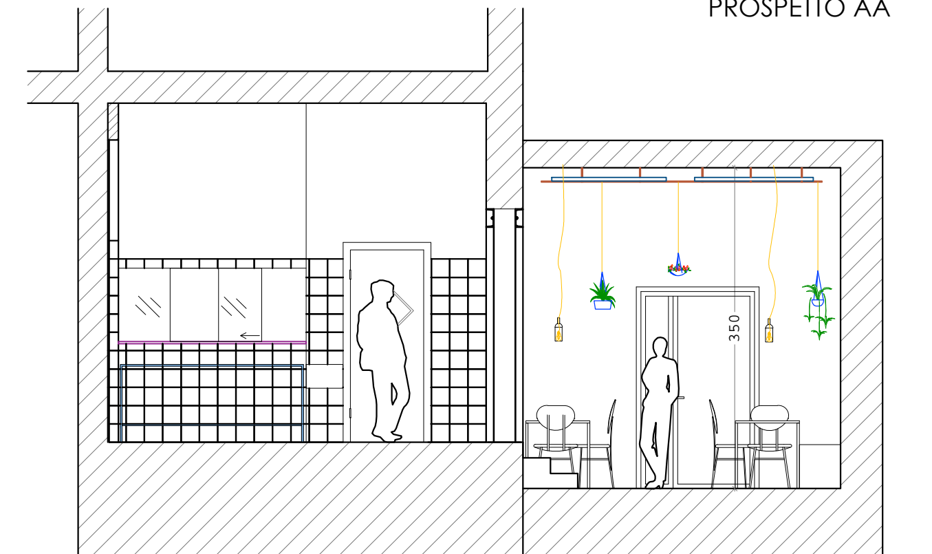
PROSPETTO CC
